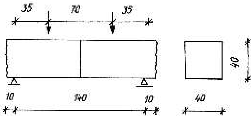
Obr. 6 Zatěžovací schéma pro zkoušku pevnosti lepidla v tahu za ohybu
