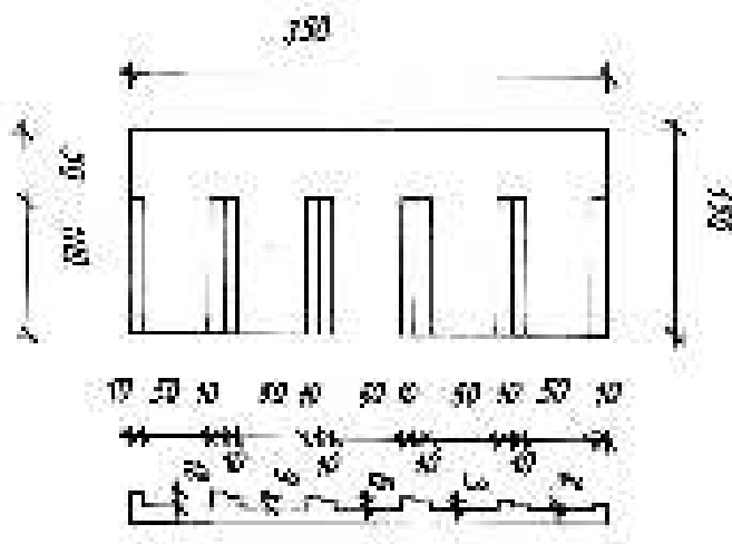
Obr. 5 Deska pro zkoušku stékavosti pojiva
